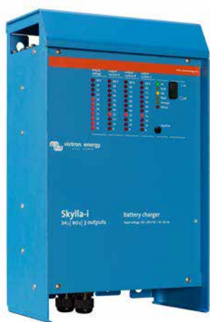
Skylla-i 24/100 (3)
